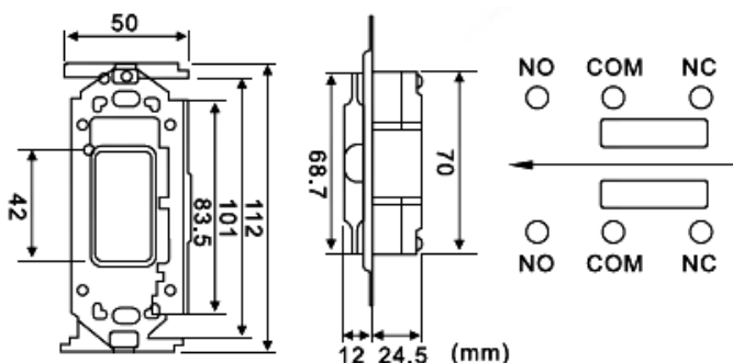
不鏽鋼面板 LK-4500AT
