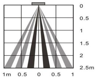
前視圖
