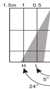
側視圖
